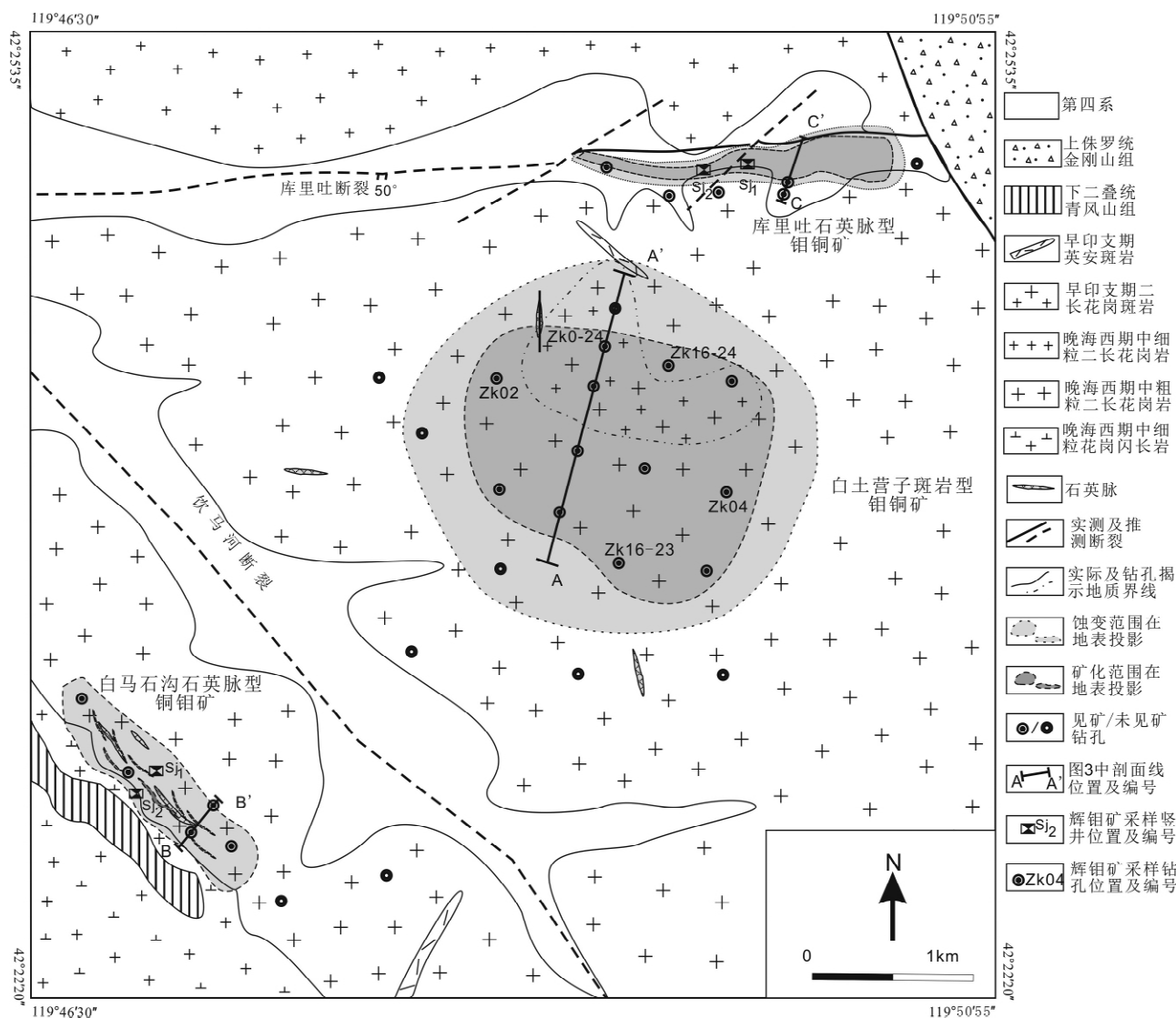
图2 白土营子钼铜矿田地质图(据朝阳金达集团实业有限公司,2006 ① ;赤峰市天恩矿业有限公司,2006 ② ;核工业 243 大队 ③ ,2010 资料修编)
