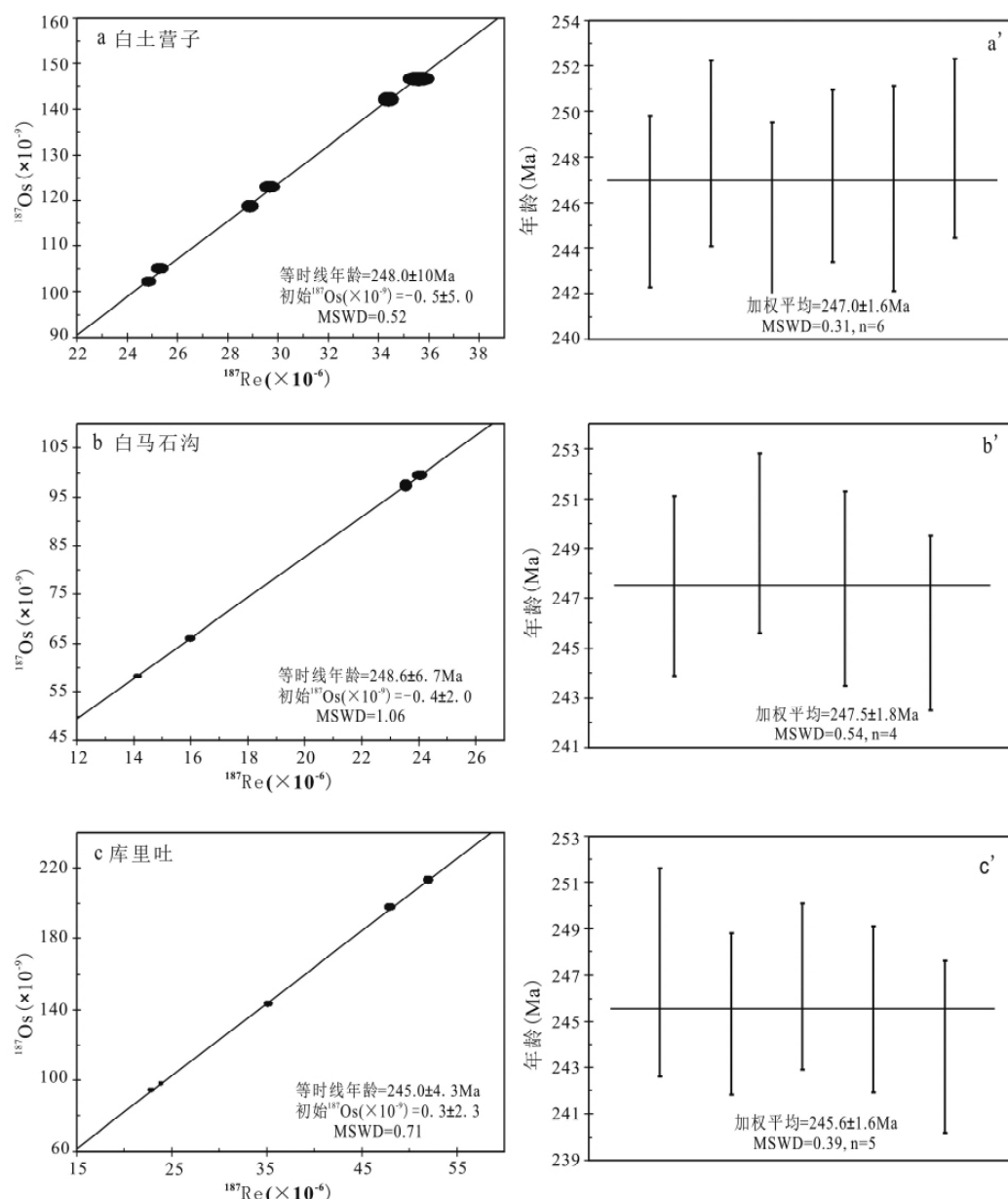
图5 白土营子斑岩型钼铜矿(a、a')、白马石沟石英脉型铜钼矿(b、b')和库里吐石英脉型钼铜矿(c、c')的辉钼矿 Re-Os 等时线年龄以及加权平均年龄
