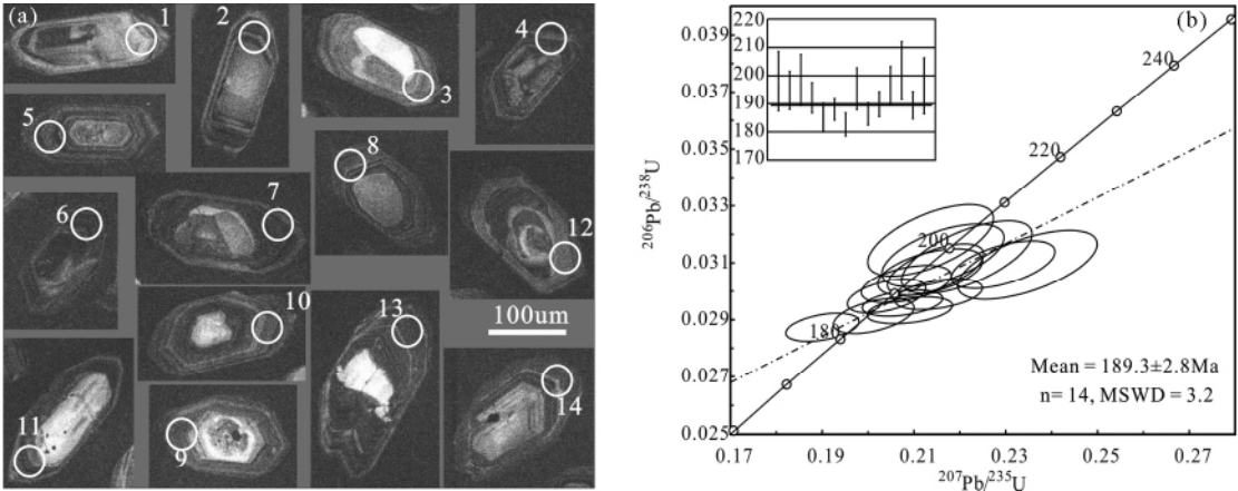
图 8 喀拉果如木二长花岗斑岩( 样品号 KL-I18) 锆石阴极发光图像( a) 和锆石 U-Pb 谐和图( b)
