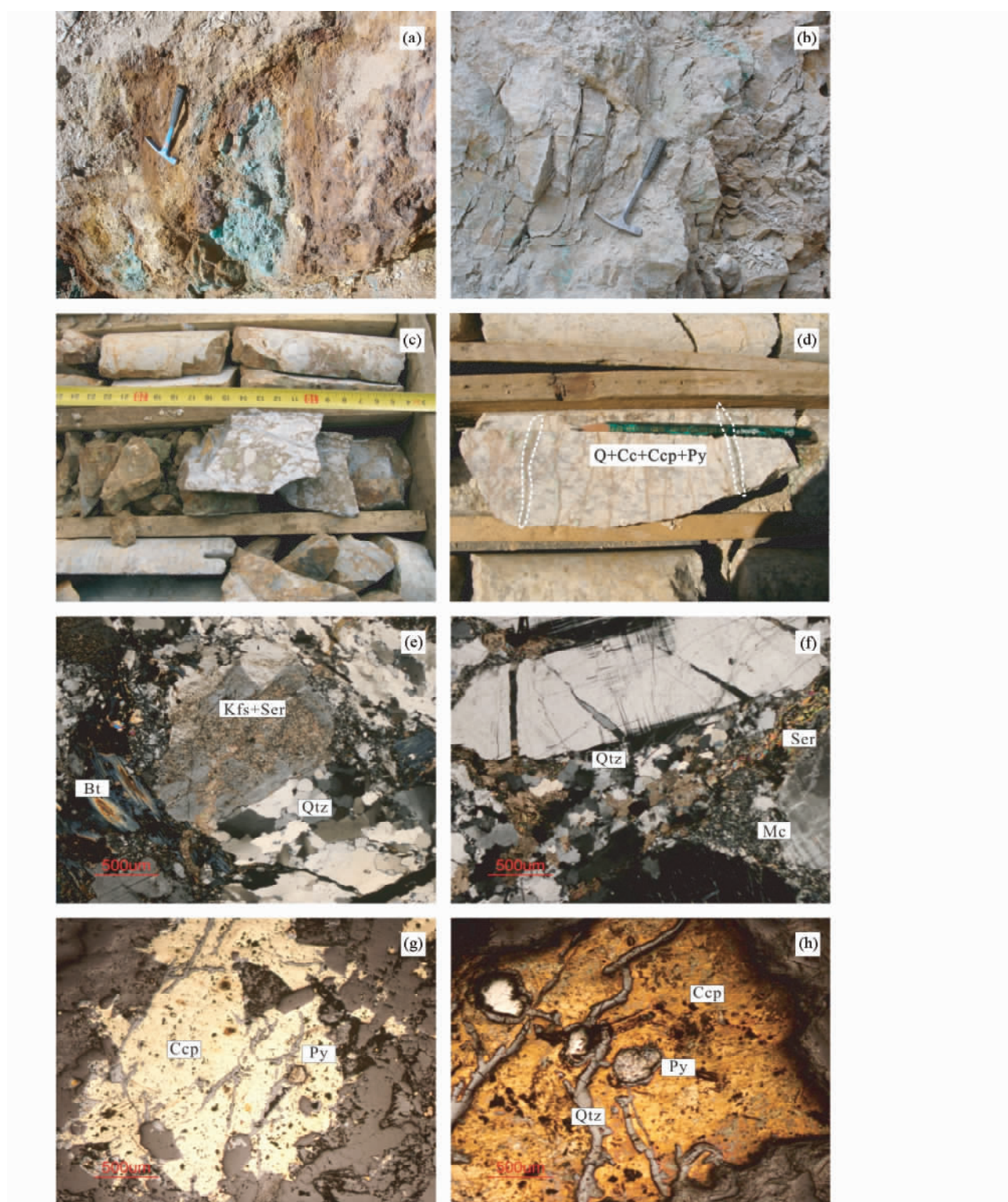
图3 喀拉果如木铜矿野外露头及显微照片
