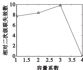
图8 容量系数对相对二次级联失效数的影响
