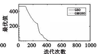
图4 函数 f_4 收敛曲线对比
