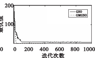
图6 函数 f_6 收敛曲线对比
