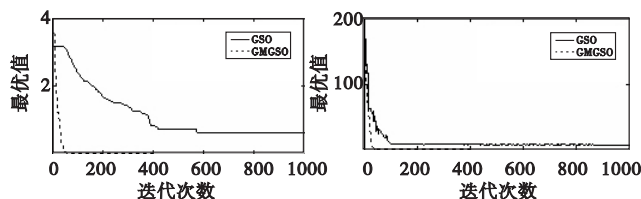
图5 函数 f_5 收敛曲线对比
