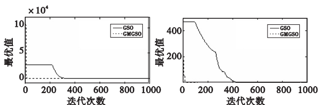
图3 函数 f_3 收敛曲线对比
