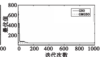
图2 函数 f_2 收敛曲线对比
