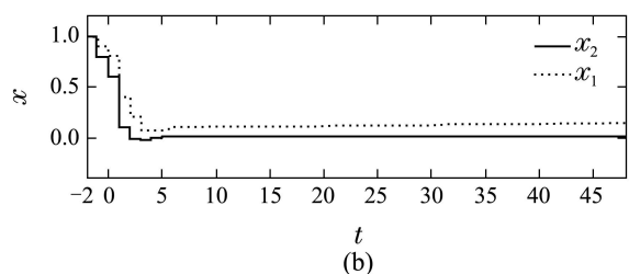
图4 控制律 K_w 下Delta算子闭环时滞系统状态轨线
