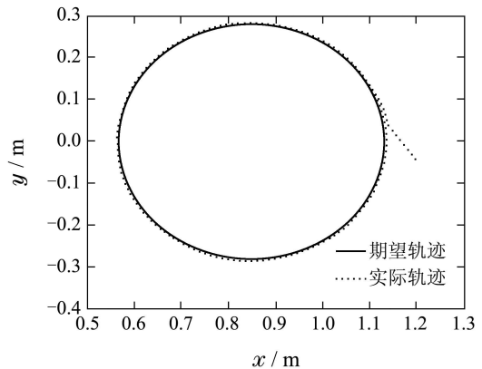
(c) 空间末端期望与实际轨迹
