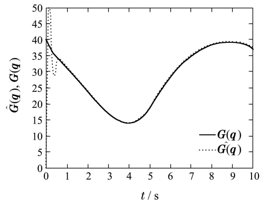
(b) 地面模型重力项 \|\mathbf{G}_x(\mathbf{q})\| 及其逼近结果
