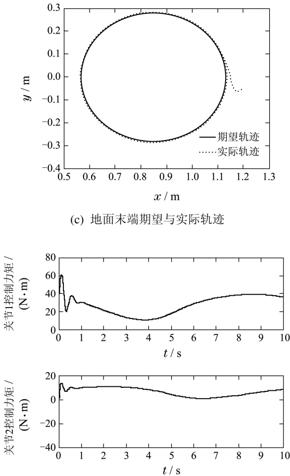
图6 地面轨迹跟踪结果
