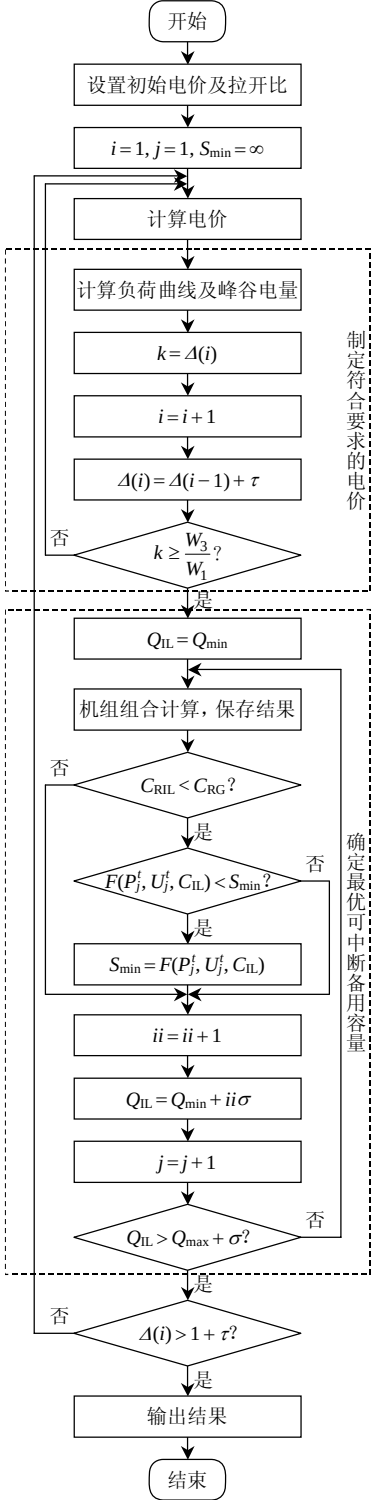
图 2 发电调度计划模型计算流程图 Fig. 2 Calculation flow chart of generation scheduling model
